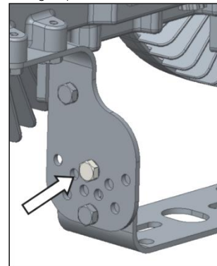
Abbildung 1 - Gelenkschraube
