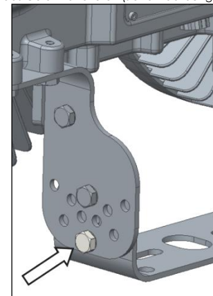
Abbildung 2 - Gelenkschraube
