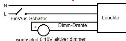
wechselnd 0-10V aktiver dimmer
