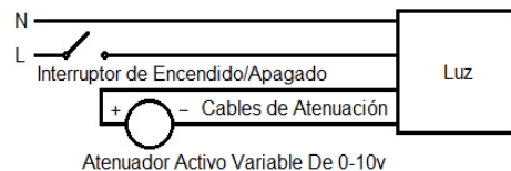
Atenuador Activo Variable De 0-10v
