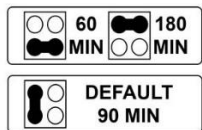
Posições do jumper de configuração da bateria
