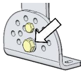
Par de apriete = 34 N-m (25 ft-lb)
